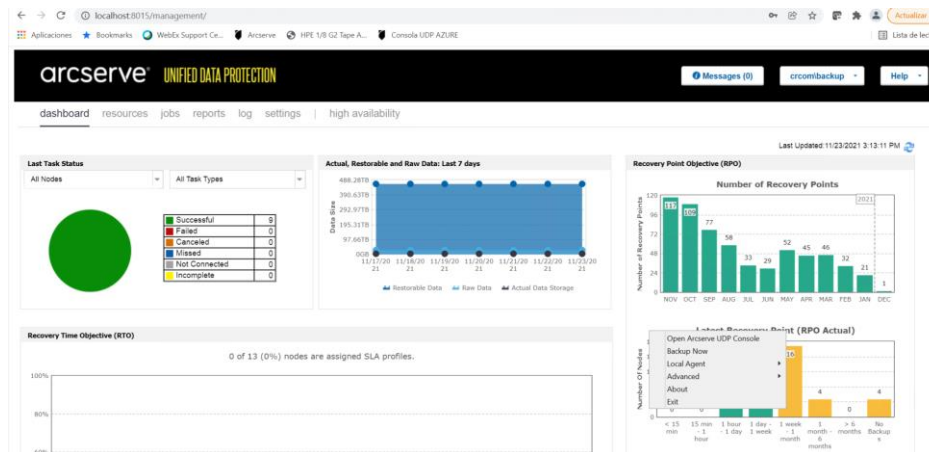
Ilustración 31 – Consolas Backup
