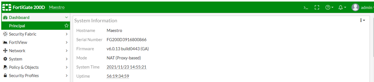
Ilustración 29 – Firewall
